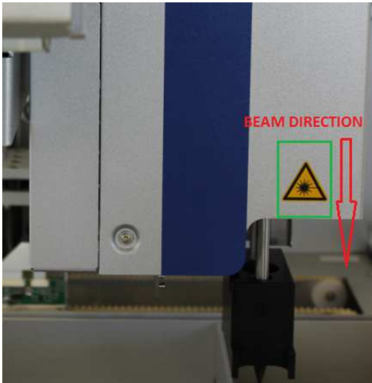
† Положение 2 для знака, предупреждающего о лазерном излучении (SP).
